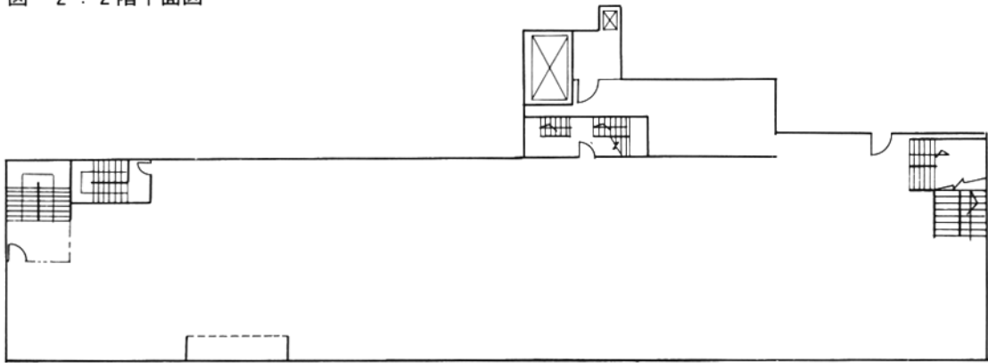
図-2 : 2階平面図
