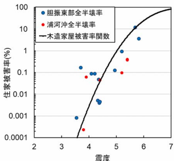
図7 1982年浦河沖地震と2018年北海道胆振東部地震の住家被害率の比較
